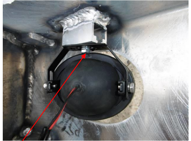
M6 bolt
